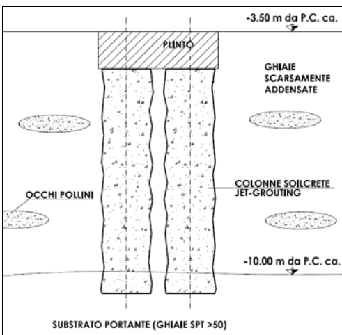
▲ Sezione tipo
