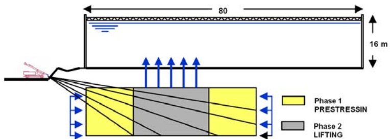
▲ Sezione schematica intervento
