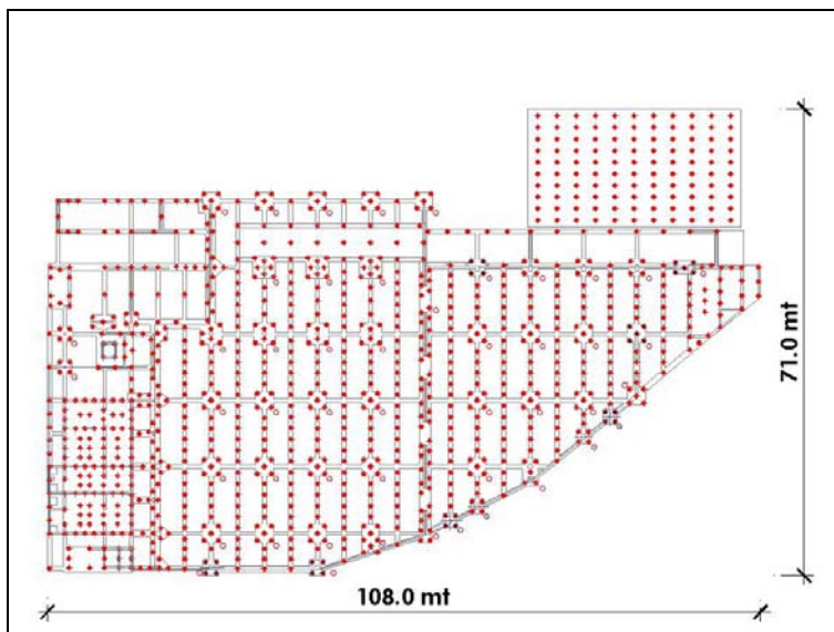
▲ Pianta dell'intervento su un'area di circa 5200 mq
